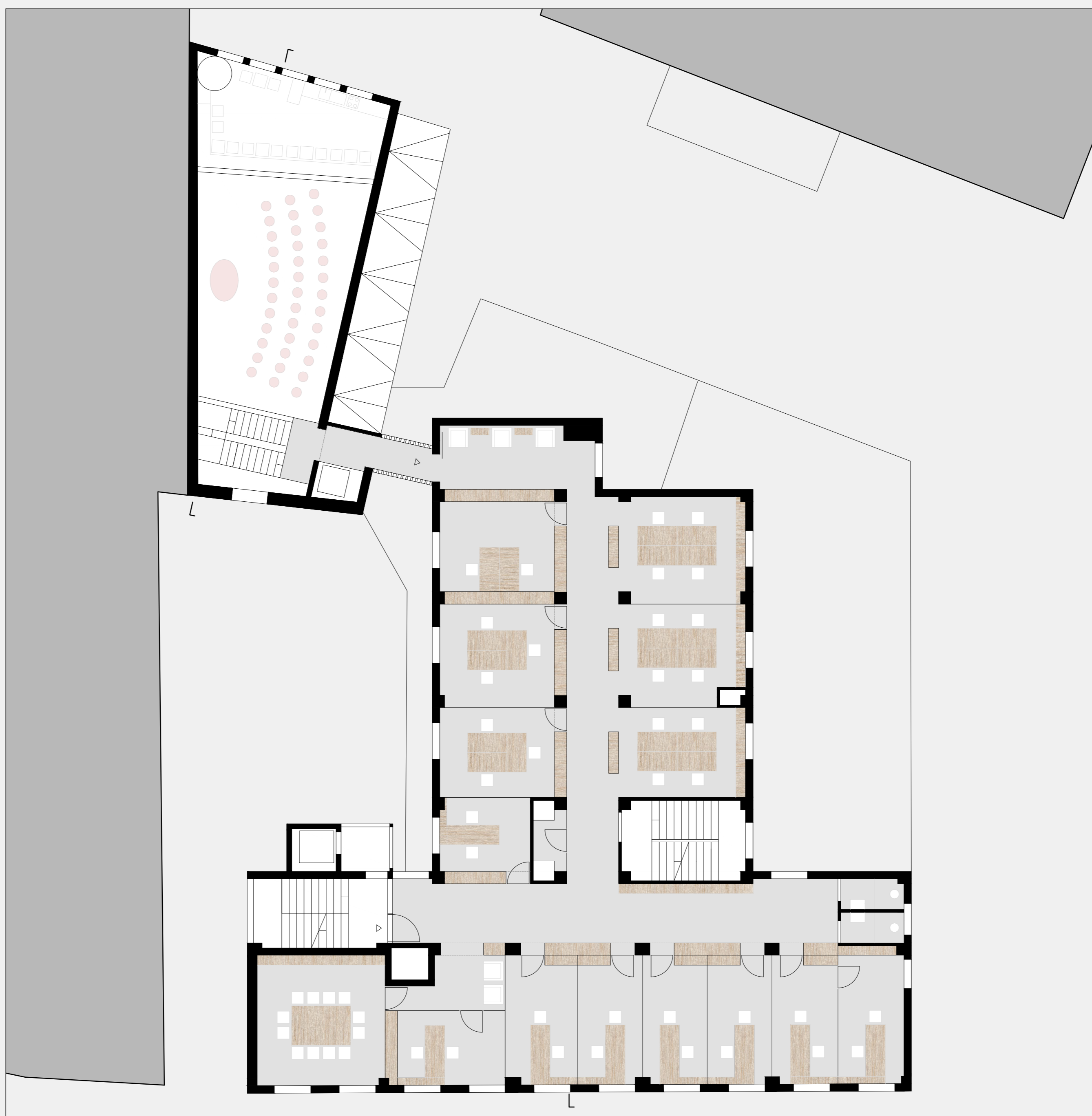
⊗ 2.OBERGESCHOSS | PIANO SECONDO
